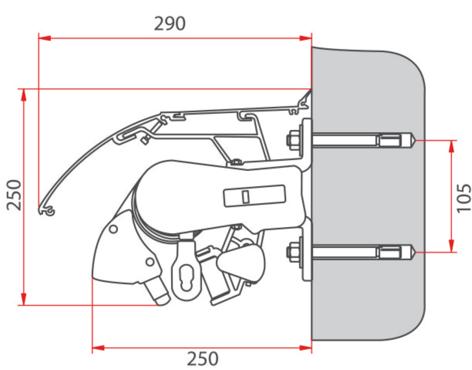
installazione parete
