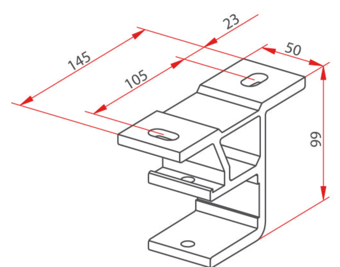
supporto soffitto
